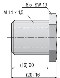
Einbaunippel für Ø 8,5 Threaded nipple for Ø 8,5
