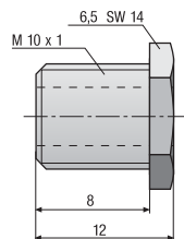
Einbaunippel für Ø 6,5 Threaded nipple for Ø 6,5
